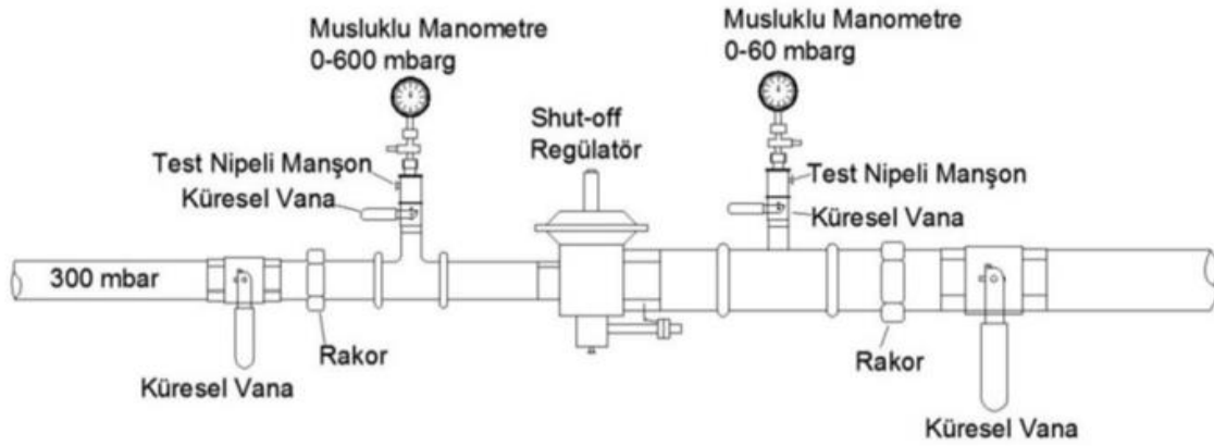
Domestik Regülatör Bağlantı Detayı
