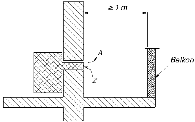
Baca Çıkışı Karşısındaki Yapı Elemanına Göre Denge Bacalı Cihazların Yerleşimi
